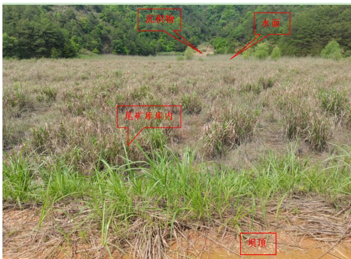
图 2-2 尾矿库现状图（坝上看向库尾）
