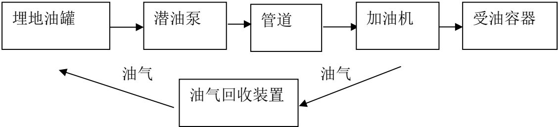
图 2.6-2 汽油加油工艺流程图
