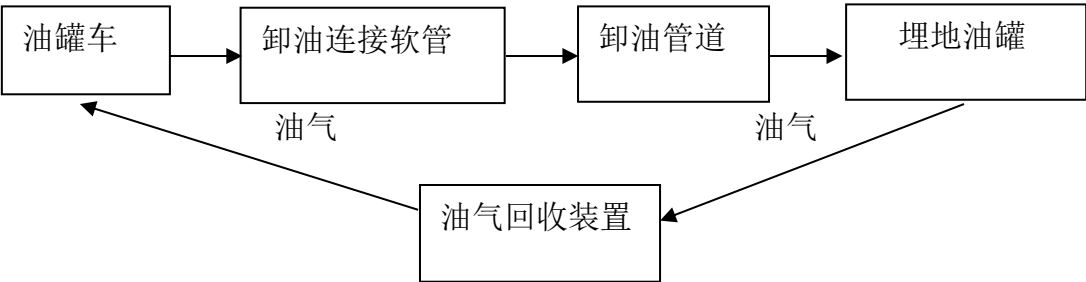
图 2.6-1 汽油卸油工艺流程图
