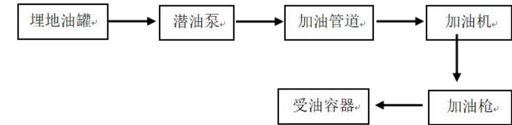
柴油加油机加油工艺，流程图如下：
