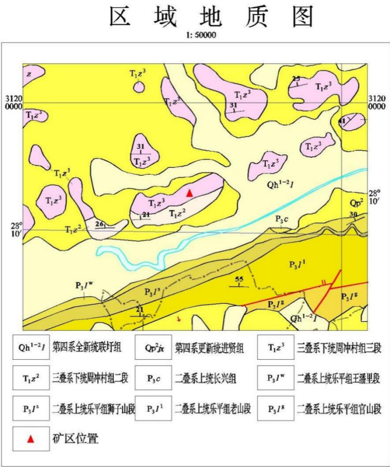
图2-2 区域地质图
