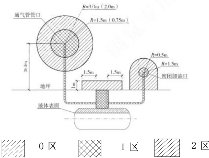
图3.5-1 埋地卧式汽油储罐爆炸危险区域划分
