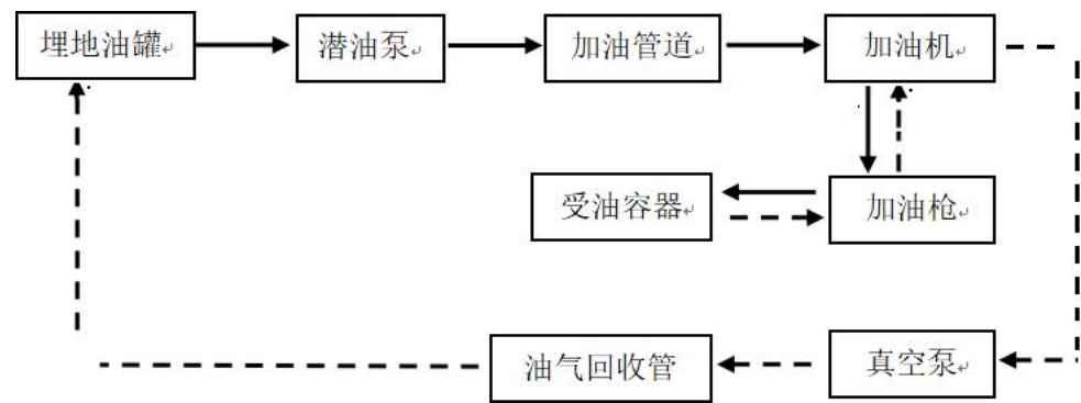
柴油加油机加油工艺，流程图如下：
