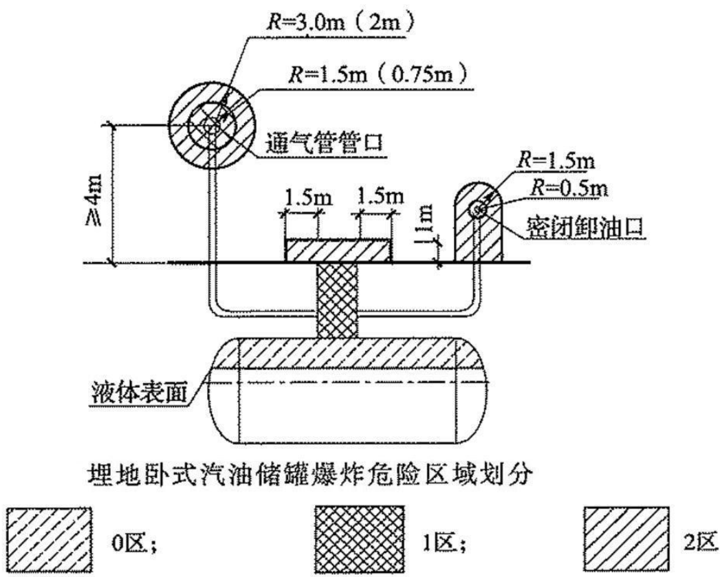
附图 3.5-2 埋地卧式汽油储罐爆炸危险区域划分图
