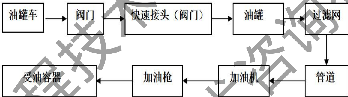
图 2.6-3 柴油卸油、加油工艺流程图
