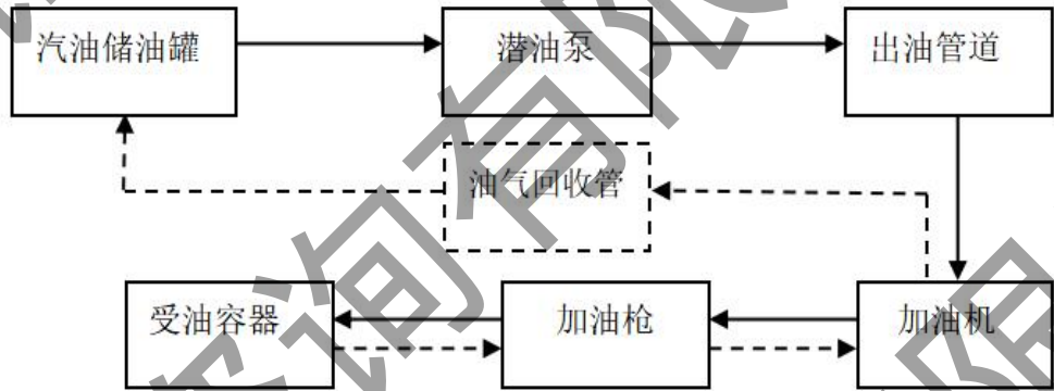
图 2.6-2 汽油加油油气回收工艺流程图
