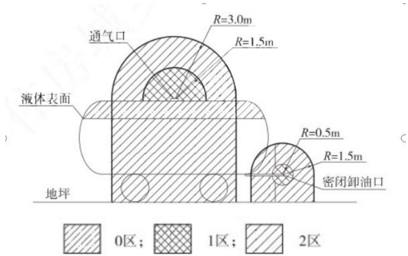
图 3.5-2 汽油储油罐车爆炸危险区域划分
