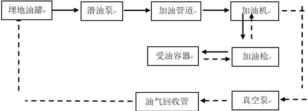
柴油加油机加油工艺，流程图如下：
