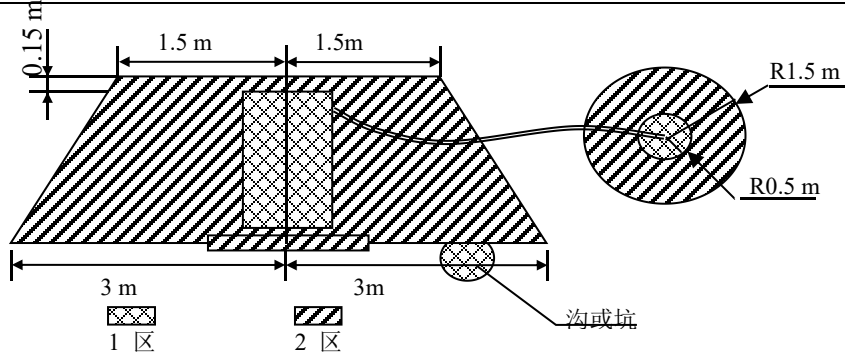
图 3-2 室外加油机危险区域分布图
