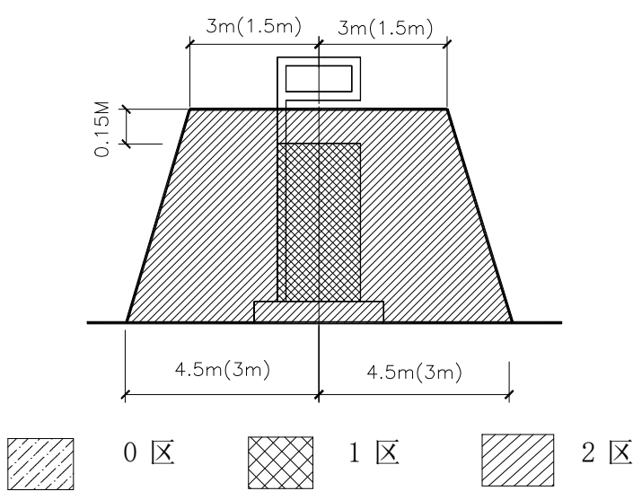
图 3.5-3 汽油加油机爆炸危险区域划分
