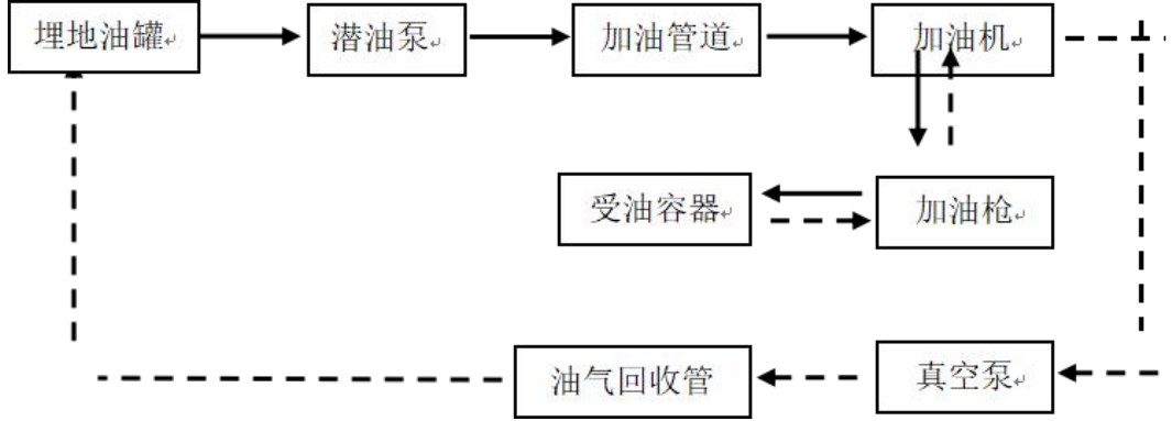
柴油加油机加油工艺，流程图如下：
