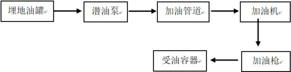
柴油加油机加油工艺，流程图如下：
