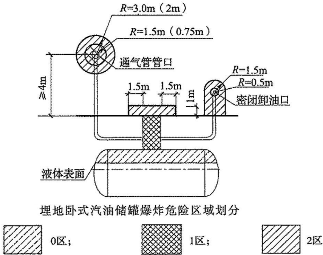
附图 3.3-2 埋地卧式汽油储罐爆炸危险区域划分图
