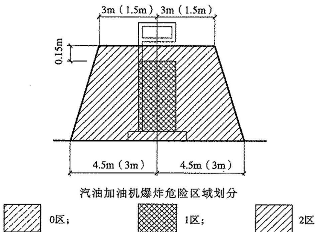
附图 3.35-1 汽油加油机爆炸危险区域划分图
