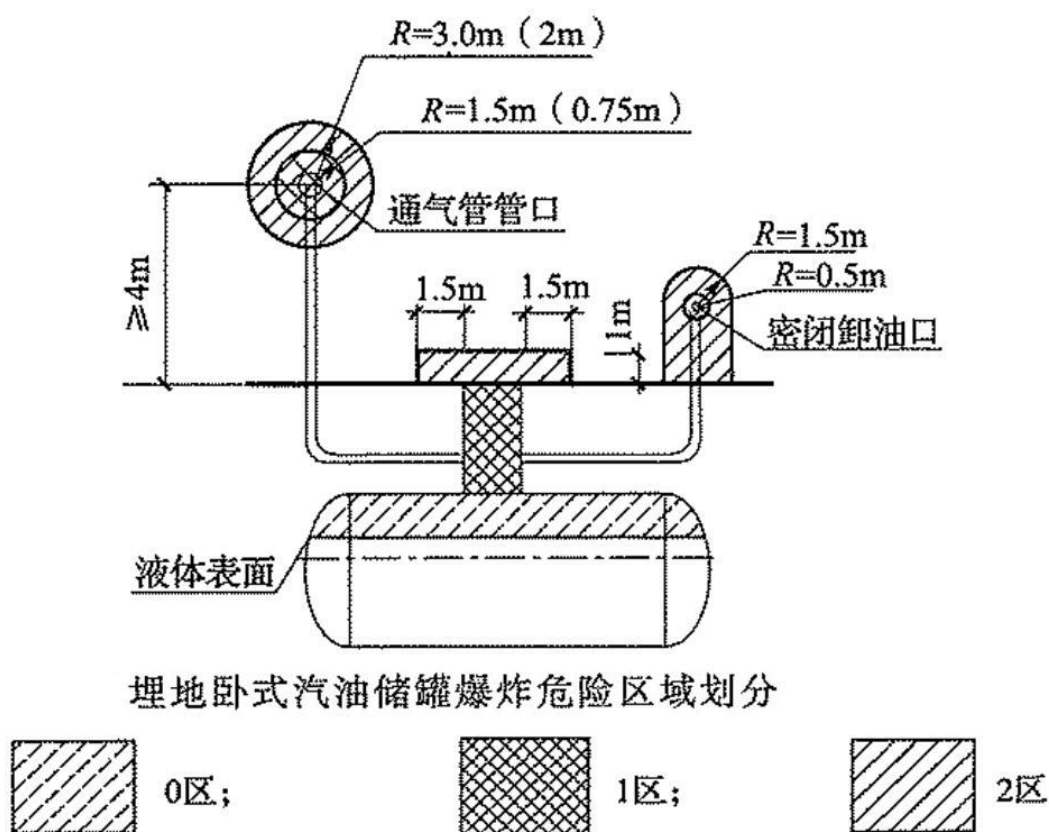
图 2.5-2.埋地卧式汽油储罐爆炸危险区域划分图
