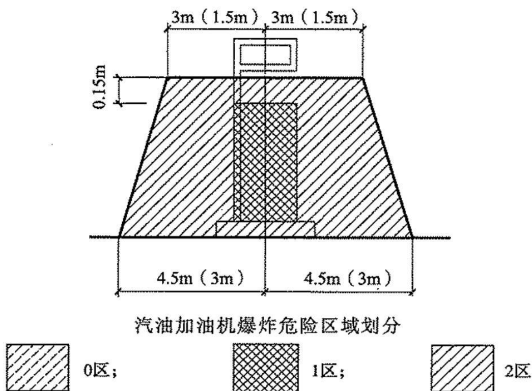
图 2.5-1.汽油加油机爆炸危险区域划分图
