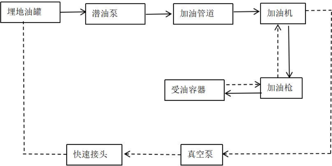
柴油加油机加油工艺，流程图如下：
