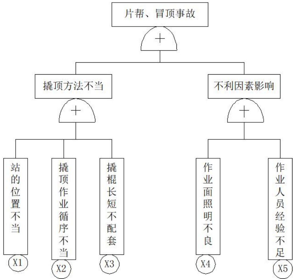
图 5.2-1 敲帮问顶片帮冒顶事故树
