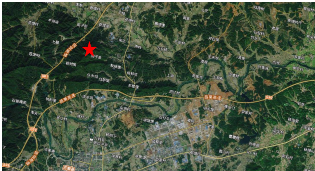
图 2-1 矿区交通位置图
