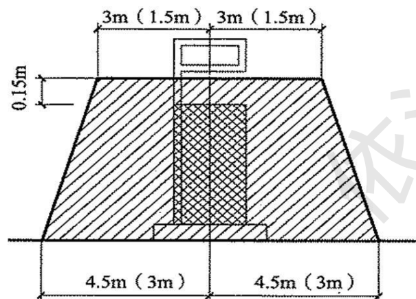
汽油加油机爆炸危险区域划分
