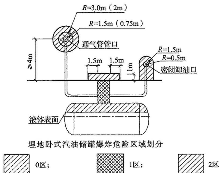
图 3.6-2 埋地卧式汽油儲罐爆炸危險區域划分圖
